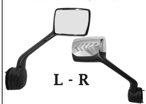
Espejo Lateral de Cofre "Cromo" con Direccional y Cuartos de 5 Flechas para Kenworth No. de Item: CNKWN307L5 / CNKWN307R5
